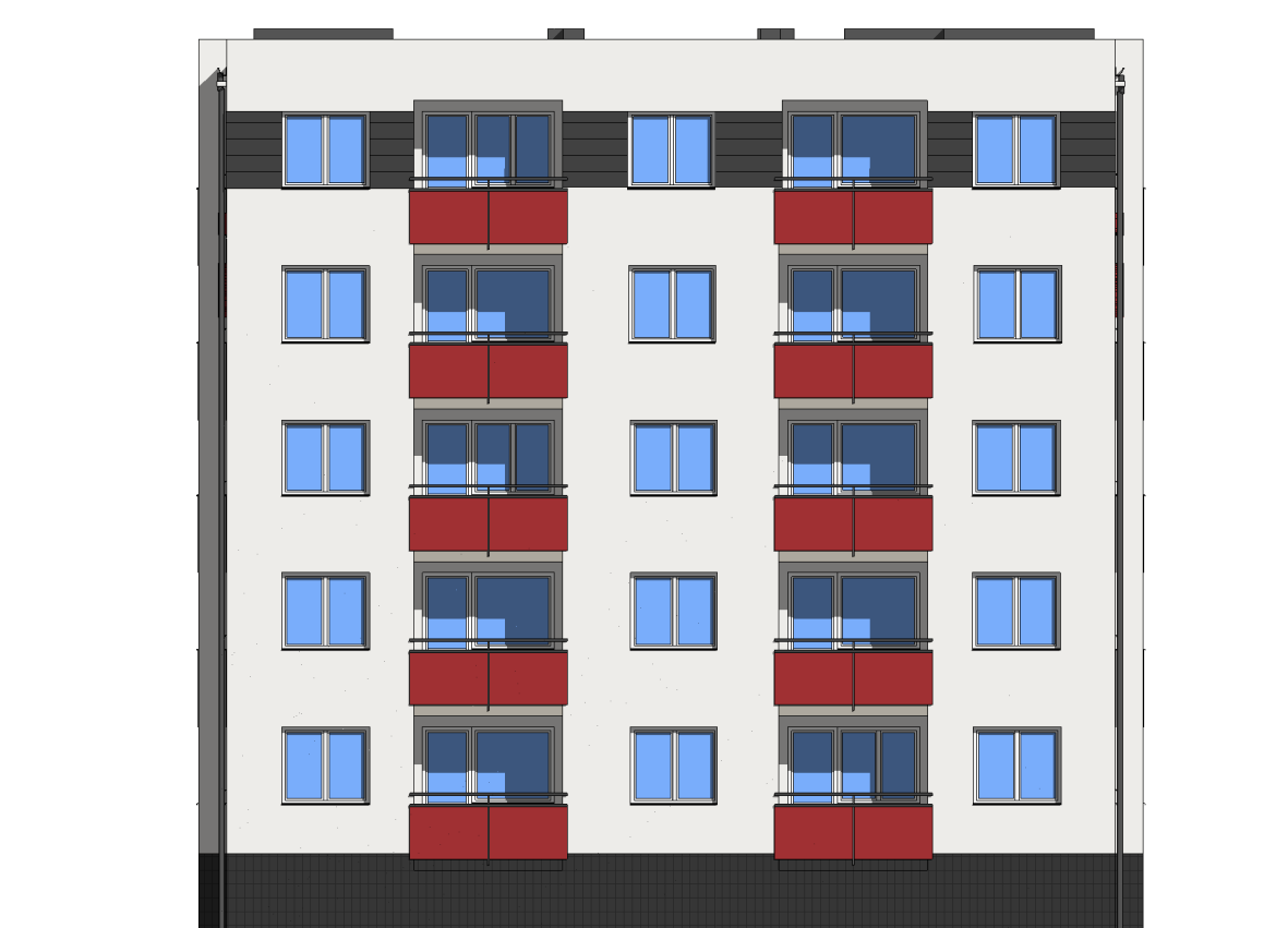
ELEWACJA POŁUDNIOWA
